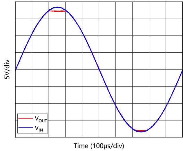
图 20. 无相位反转
