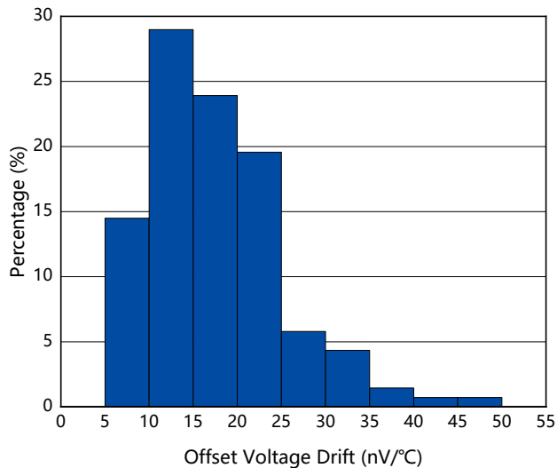
图 2. 失调电压温漂分布
