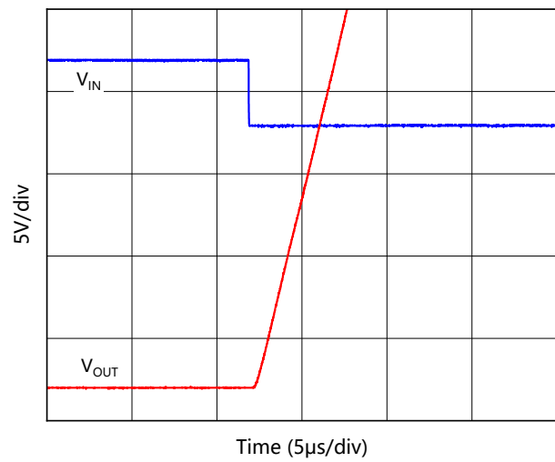
图 22. 负过载恢复
