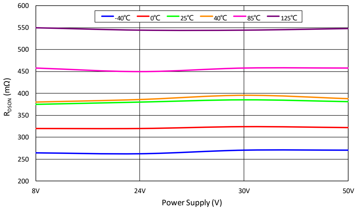
图 4. R_{DS(on)} VS. 电源电压
