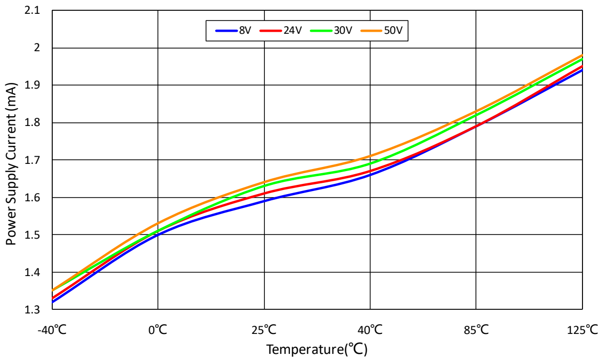
图 2. 电源电流 vs. 温度
