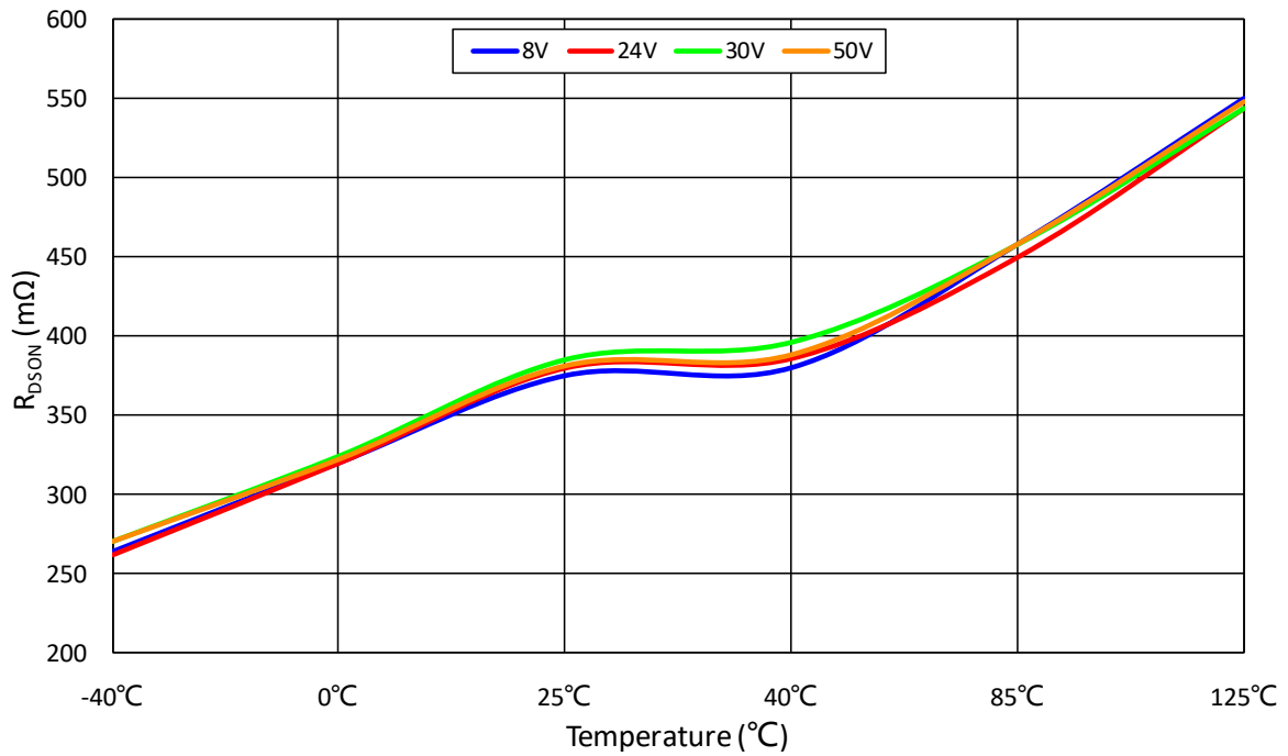
图 3. R_{DS(on)} VS. 温度
