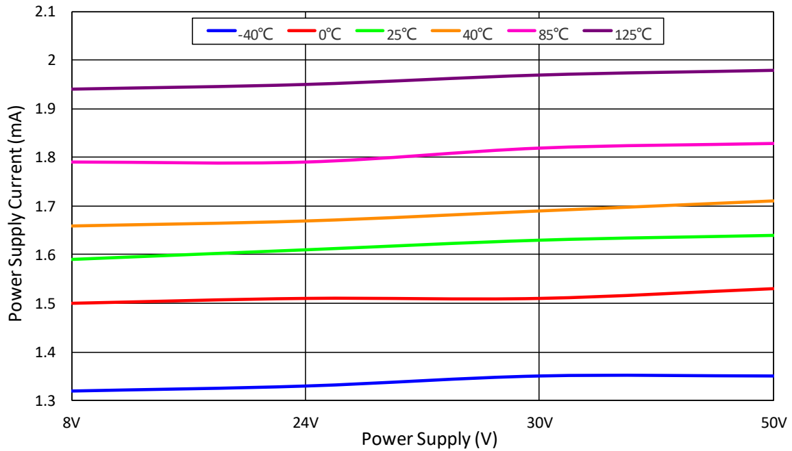
图 1. 电源电流 vs. 电源电压
