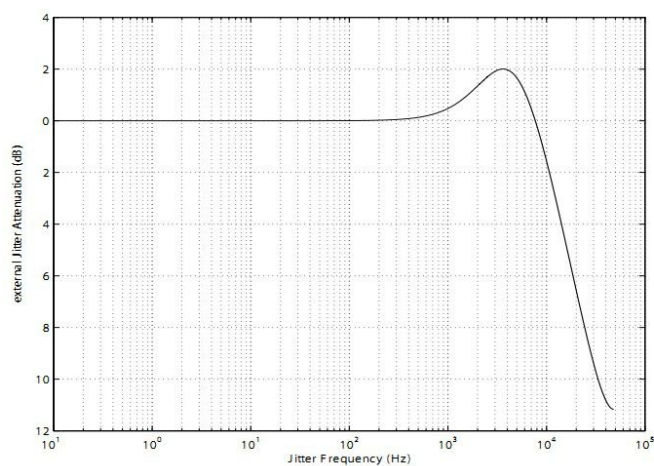
PLL的抖动衰减特性曲线
