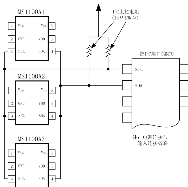
图.5 连接多个 MS1100
