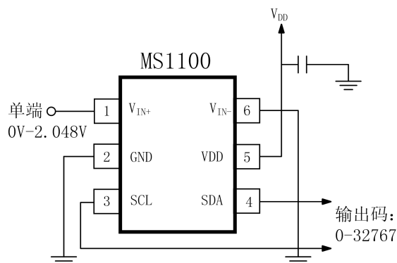
图.7 单端输入测量
