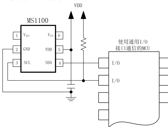
图.6 对单个 MS1100 使用通用 IO 口
