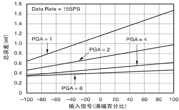
总误差 vs 输入信号
