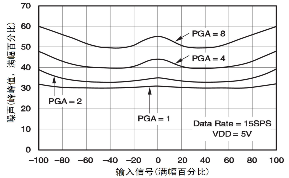
噪声 vs 输入信号
