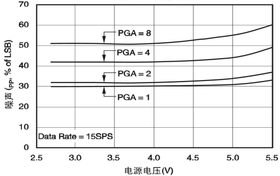
噪声 vs 电源电压
