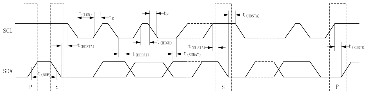
图.1 I^2C 时序图
