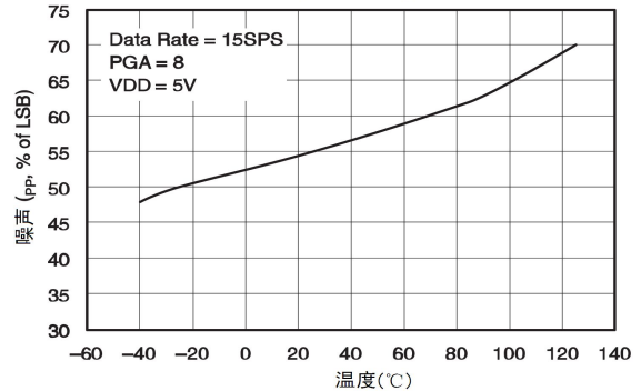
噪声 vs 温度
