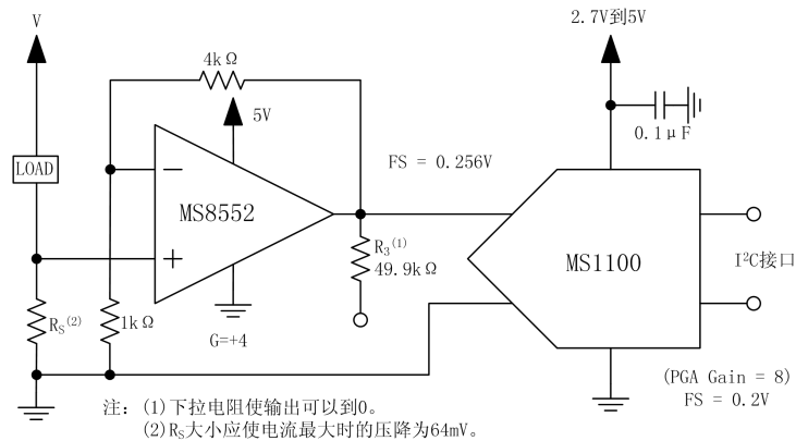
图.8 低端电流测量
