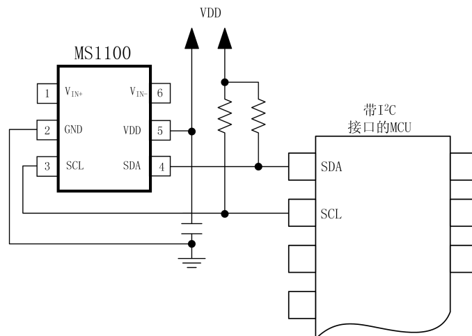
图.4 MS1100 的典型连接方法
