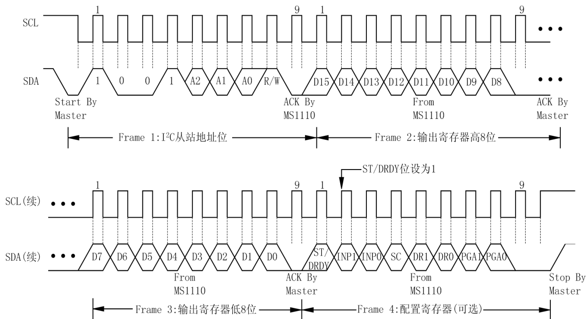
图.2 MS1100 的读操作时序图
